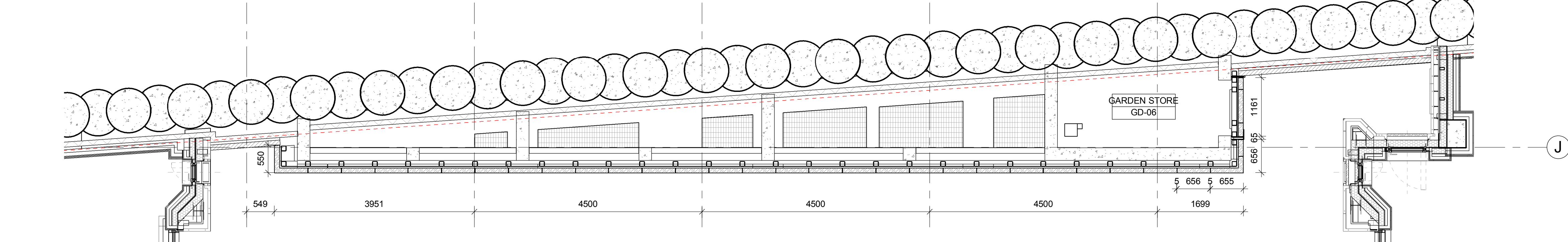
3 Garden Level Plan 1 : 50
